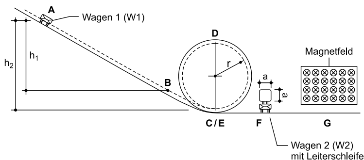
Abb. 1: (Seitenansicht der Anordnung, nicht maßstäblich)
