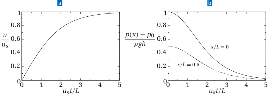
Abb. 4.11: Instationärer Ausfluß durch ein horizontales Rohr der Länge L . a Geschwindigkeitsentwicklung nach einem plötzlichen Öffnen. b Zeitliche Entwicklung des Drucks am Einlaß des Rohres ( x/L = 0 ) und in der Mitte ( x/L = 0.5 ) nach dem Öffnen.
