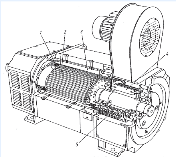
Abbildung 3.1 Aufbau einer Gleichstrommaschine (ABB)
